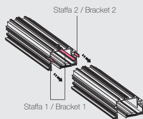
GIUNZIONI LINEARE LINEAR JUNCTIONS
